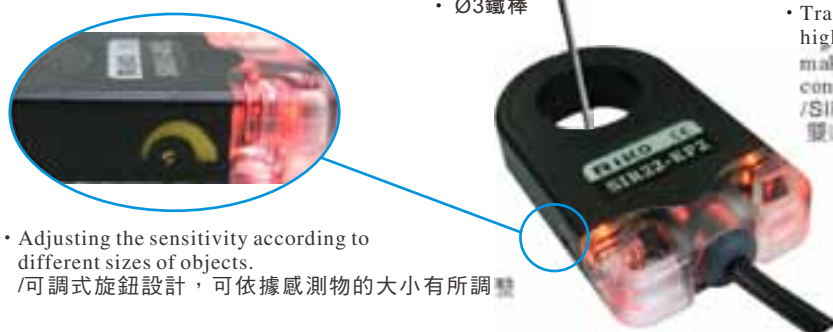
Pre-wired type / 出線式
